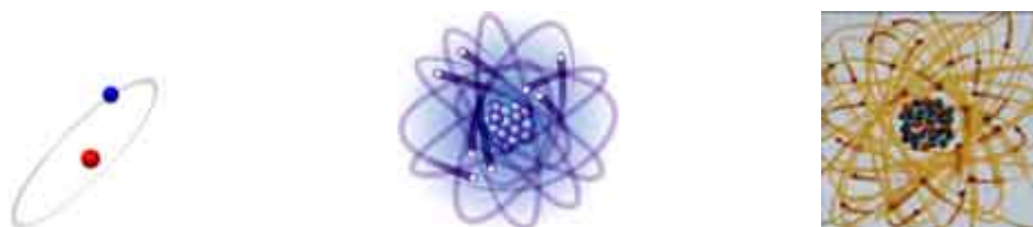
اتم اورانیوم 92 پروتون و 92 الکترون (اتم اکسیژن 8 پروتون و 8 الکترون و) اتم هیدروژن (1 پروتون و یک الکترون)
