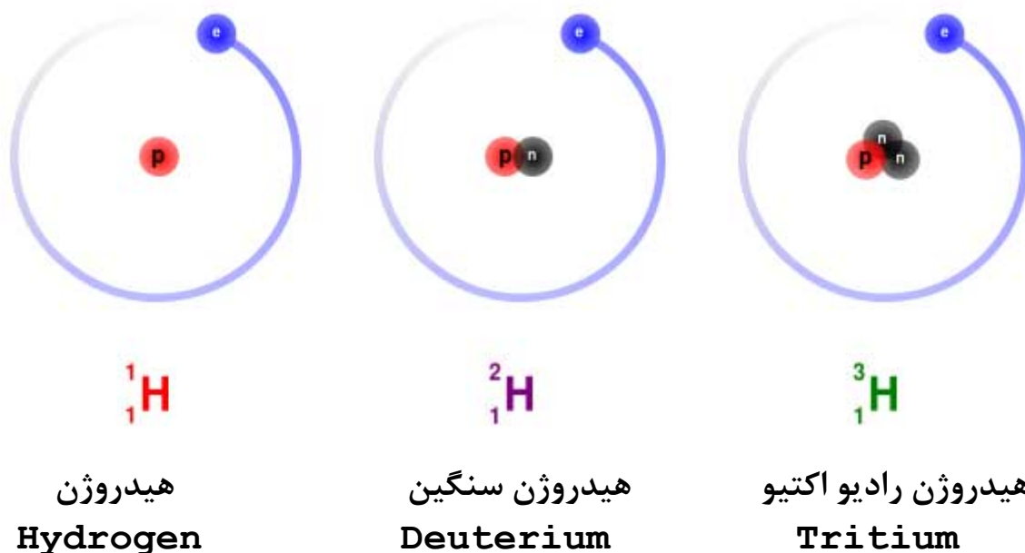
شکل (1-1) ایزوتوپهای مختلف هیدروژن.
